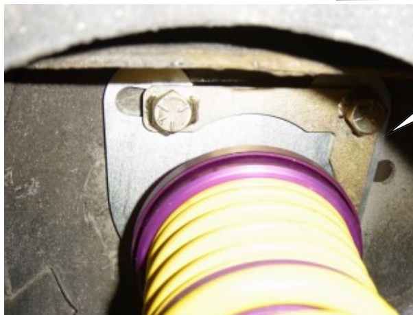
Eingebautes Federbein von unten. Installed coilover strut from below.
