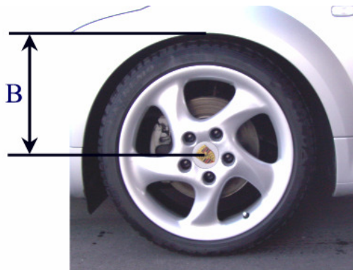
Abstandsmaß B - Radmitte—Bördele
