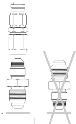
Dichtscheibe / Gasket
