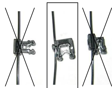
Edge Clip
