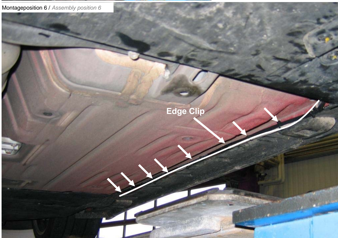
Edge Clips
